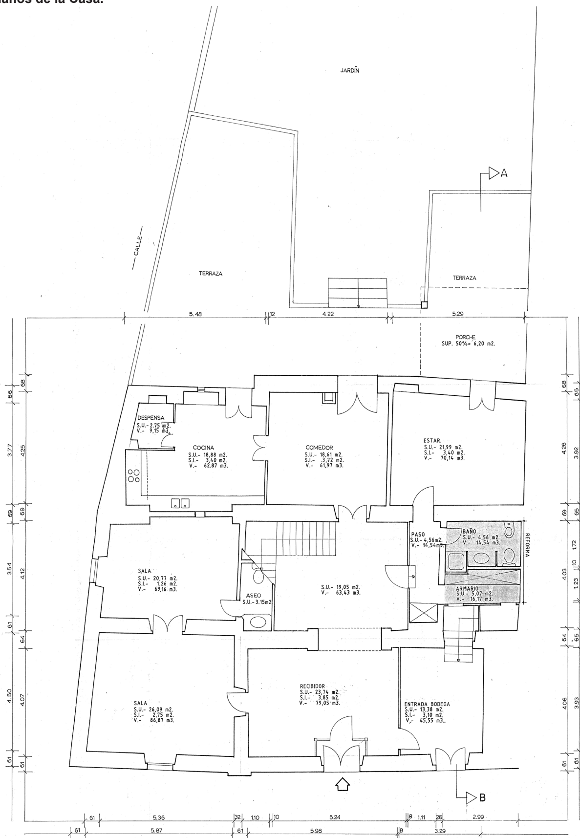
PLANTA BAJA_ SUP. CONSTRUIDA 251,45 M2 + PORCHE 12,40M2
