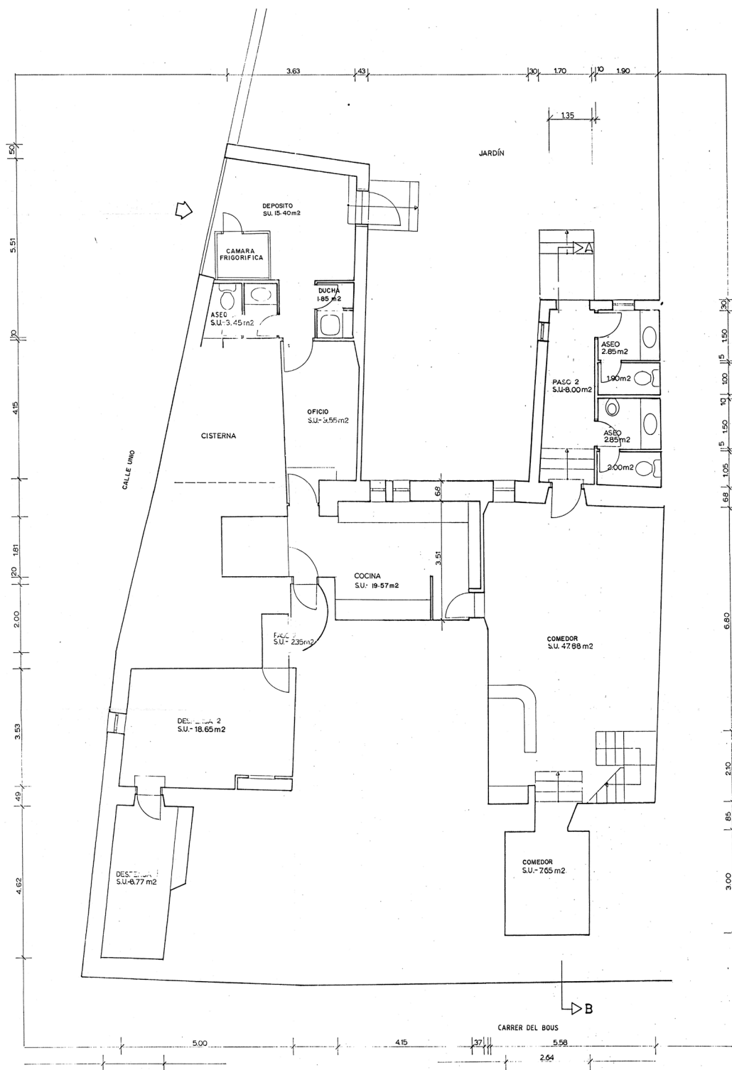
PLANTA SEMISOTANO _ SUP. CONSTRUIDA 223 M2
