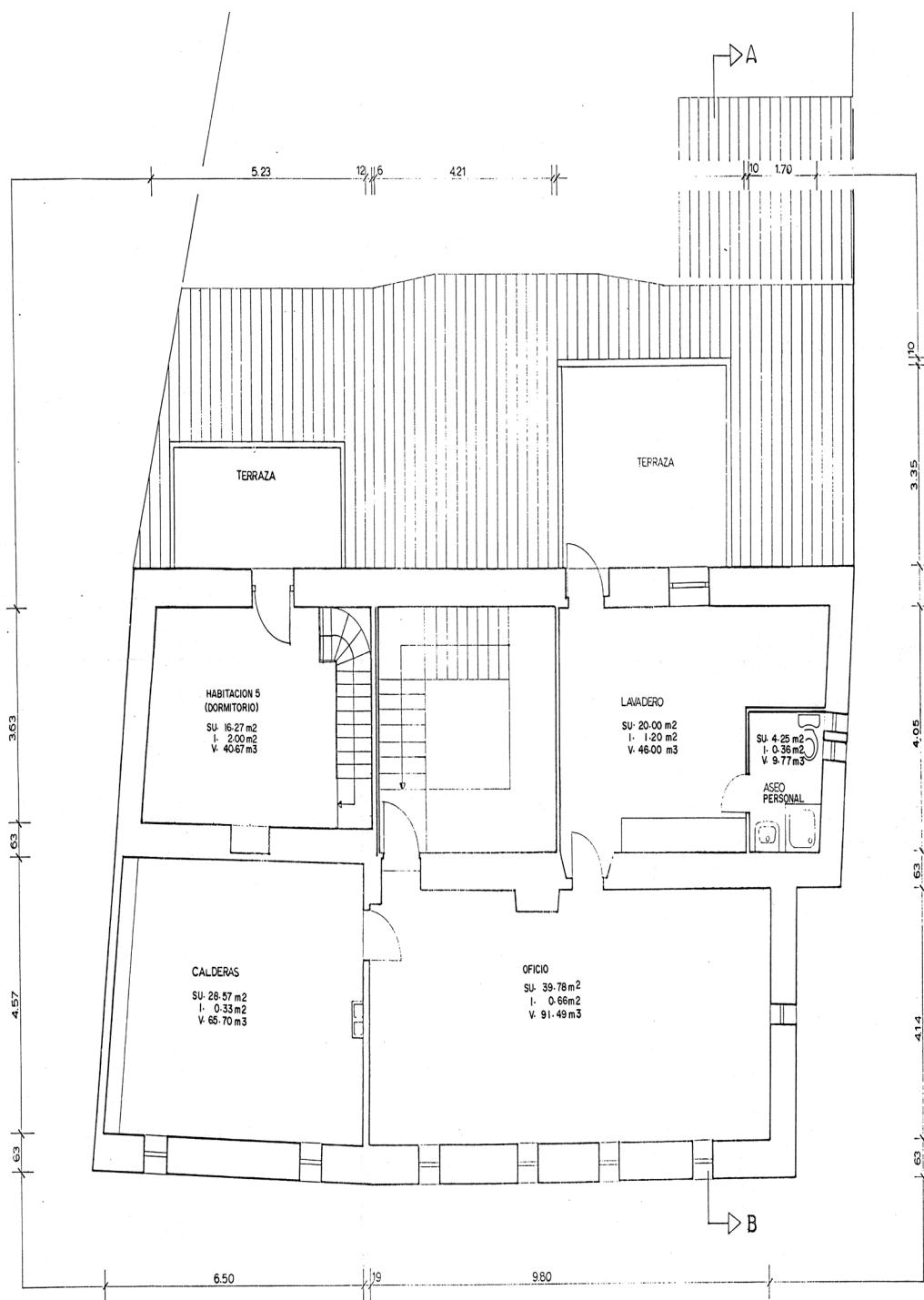
PLANTA PISO _ SUP. CONSTRUIDA 251,45 M2
